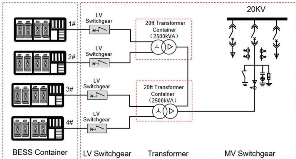
Figura 1. Schema monofilara sistem
